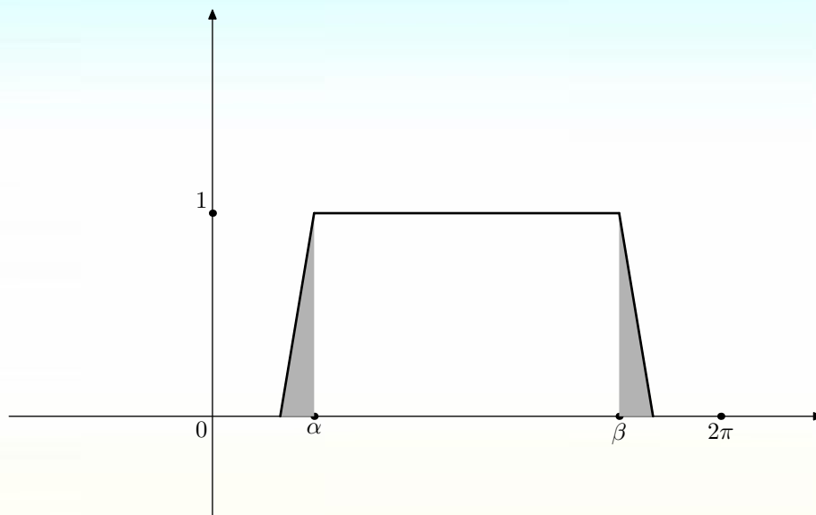
Рис. 4: Сглаживание разрывов
