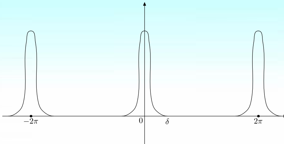
Рис. 2: Сглаживающая функция
