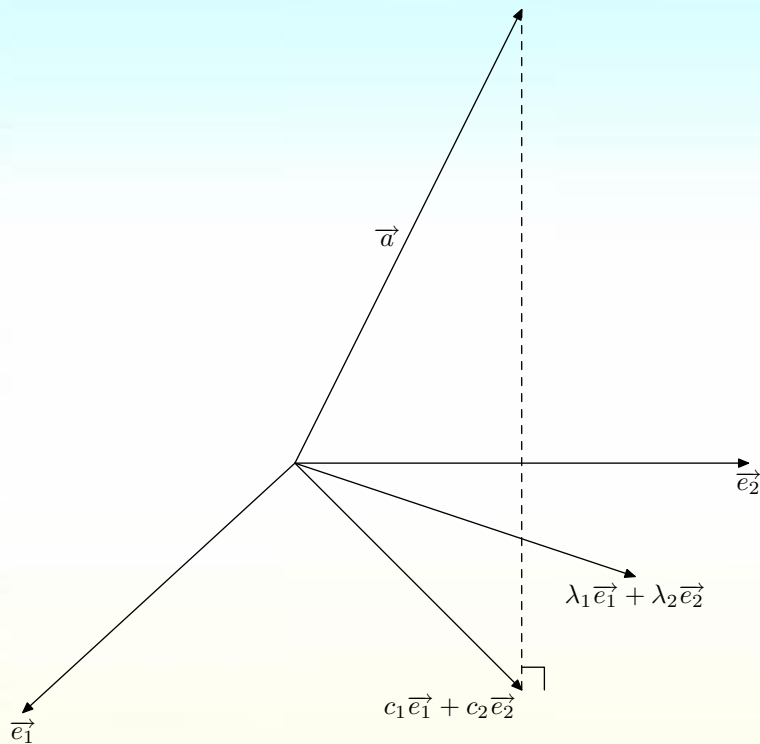
Рис. 1: Перпендикуляр — наименьшее расстояние до подпространства
